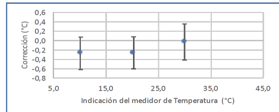
Figura 1.- Curva de Calibración del Medidor de Temperatura
