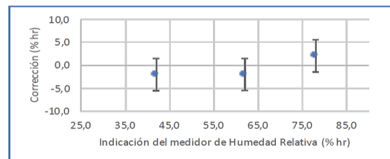
Figura 2.- Curva de Calibración de Humedad Relativa
